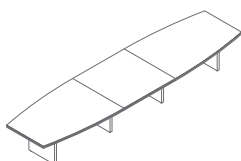
X10 5400 / 1400-1000 / 760 331.2 kg
