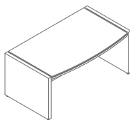
X02 1700 / 900-970 / 760 104.85 kg
