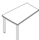
X14 600-800 / 1200 / 760 36.65 kg
